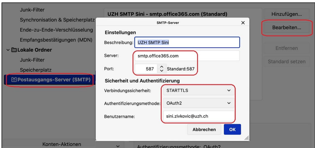
Abb 8: Kontoeinstellungen: Postausgangs-Server (SMTP)
