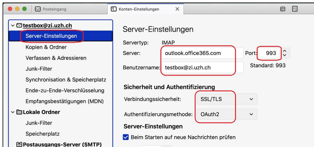
Abb 7: Kontoeinstellungen: Server-Einstellungen (IMAP)
